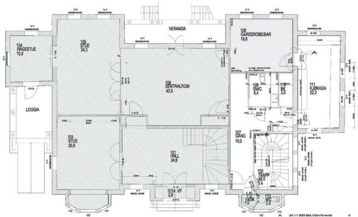
Plantegning 1. etasje. Omfang interiørfredning er markert med blå skravur.
