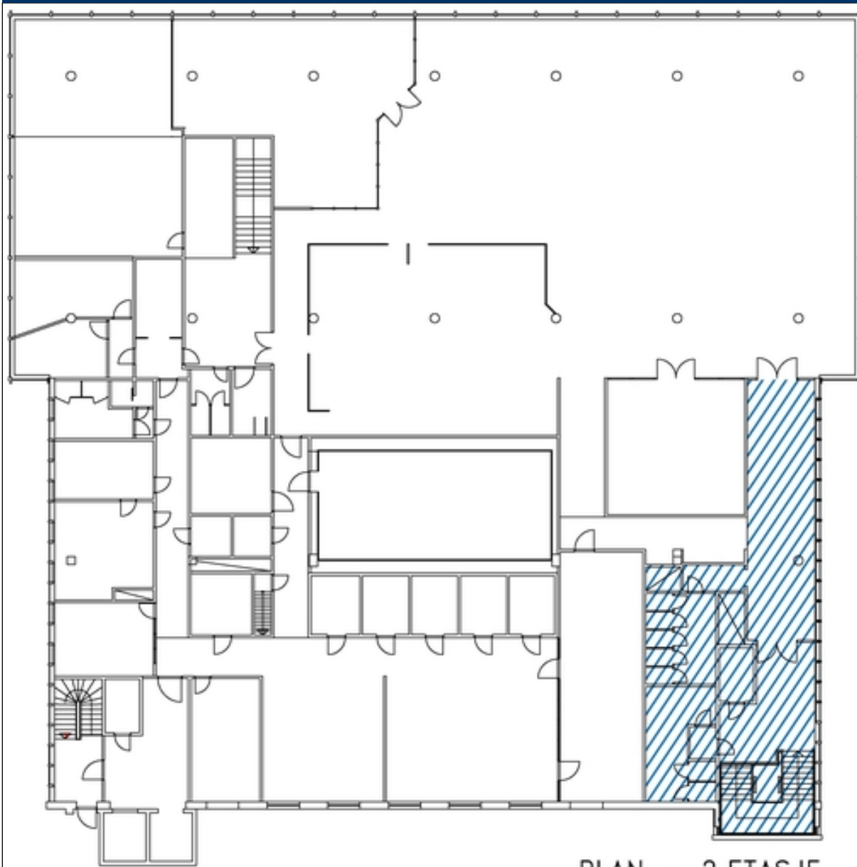
PLAN - 2. ETASJE
