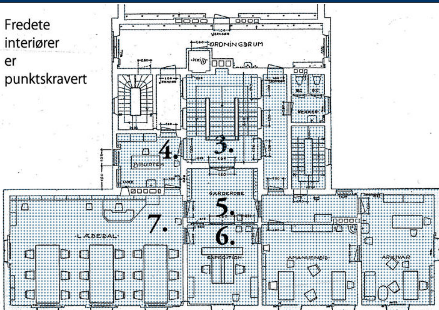
Opprinnelig plantegning 2. etasje 1924. Omfang interiørfredning er markert med blå skraver.
