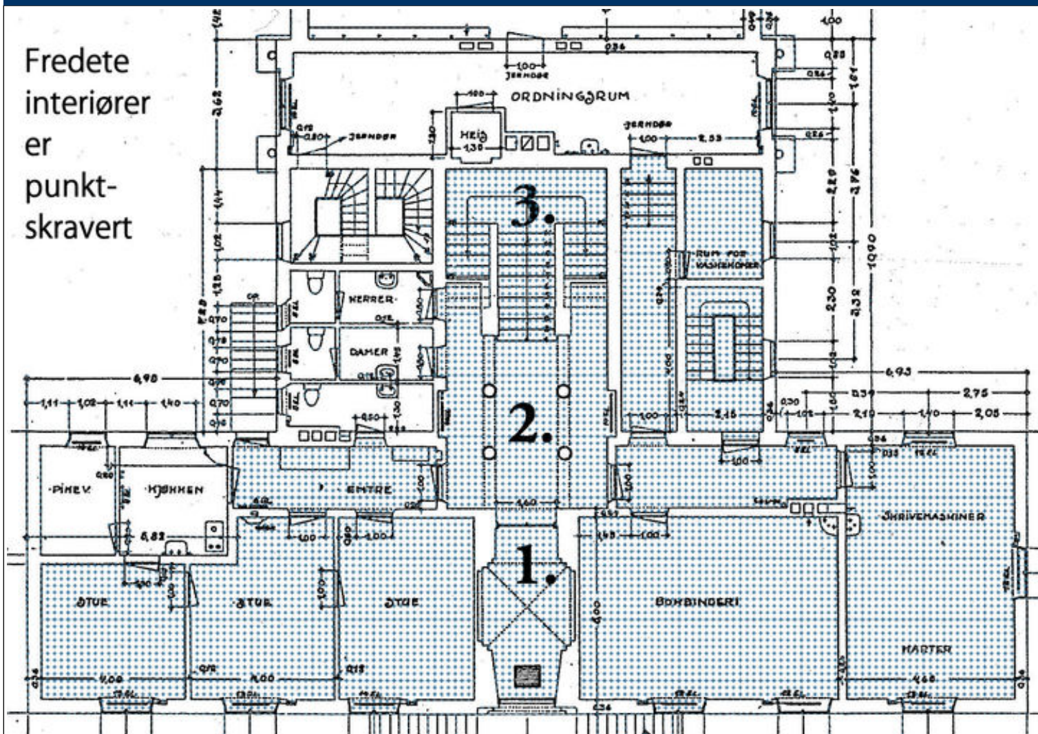
Opprinnelig plantegning 1. etasje 1924. Omfang interiørfredning er markert med blå skravur.
