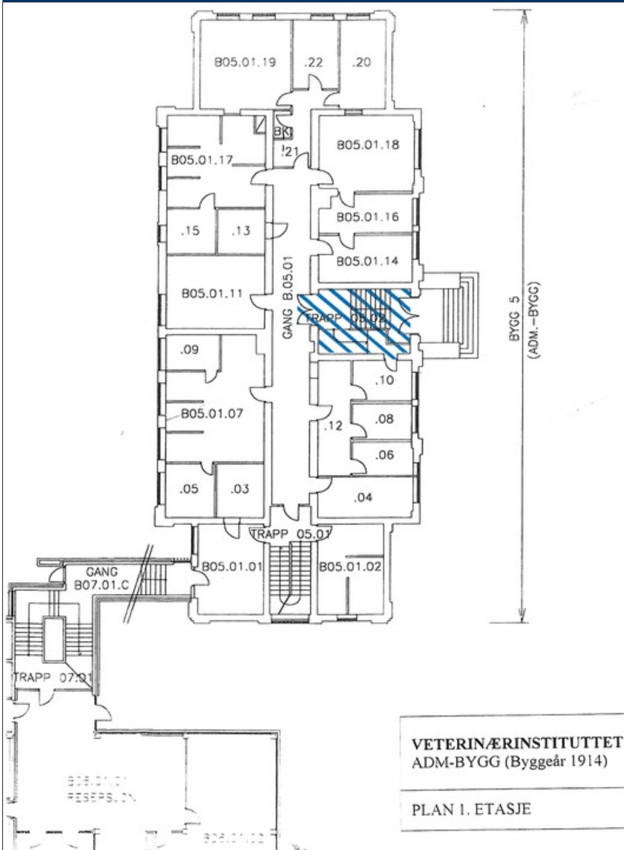
Plantegning 1. etasje, Veterinærinstituttet. Omfang interiørfredning er markert med blå skraver.
