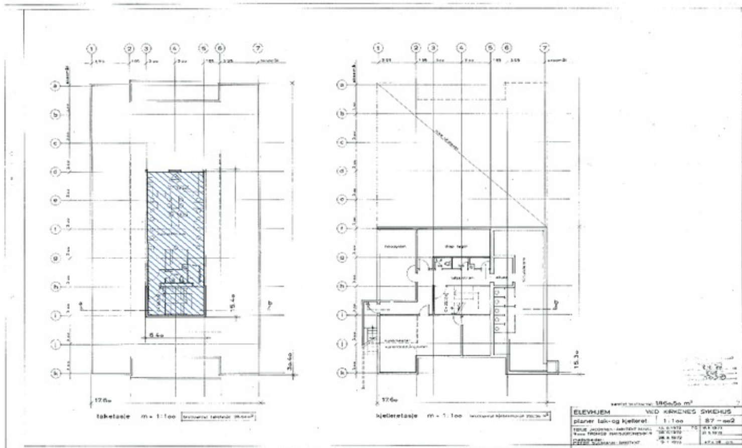
Plantegning taketasje, elevhjem. Omfang interiørfredning er markert med blå skraver.
